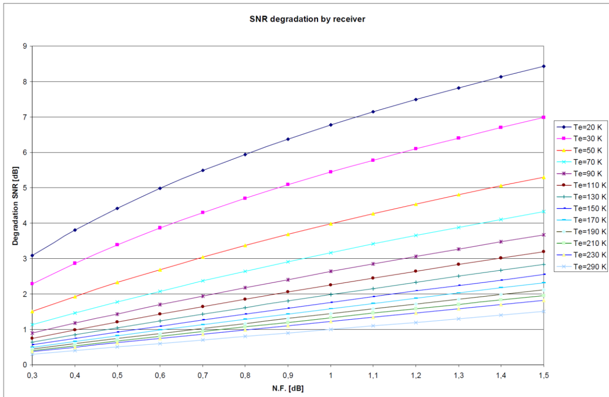
Obr. 10. Degradace SNR v závislosti na šumovém čísle přijímače. Parametrem je T_e = T_{SKY} + T_G + T_{bM} .
