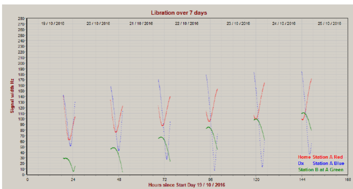
Obr. 2. Predikce rozšíření signálu během jednoho týdne. Stanice A je umístěna v ČR a stanice B v Japonsku [2].
