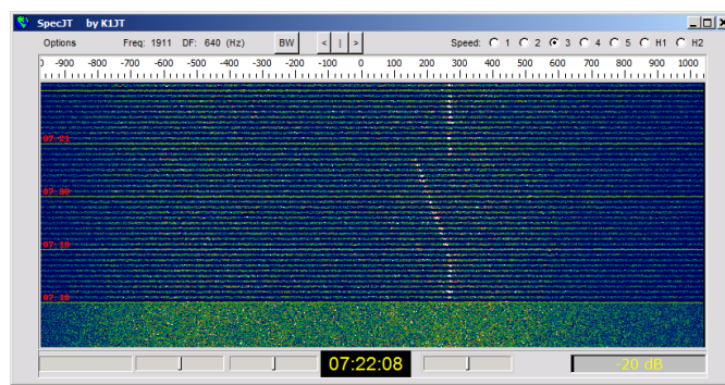
Obr. 14. Měření echa po sekvencích.
