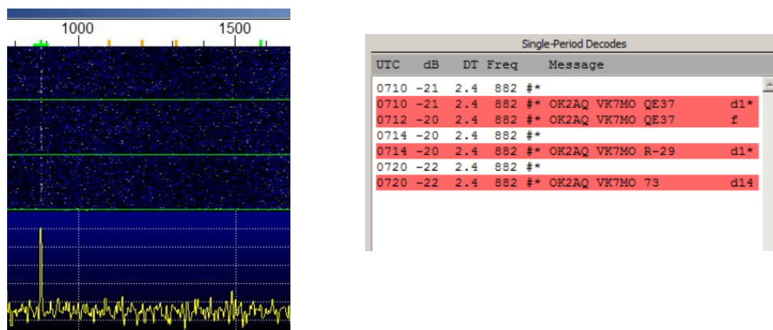
Obr. 4. Signál JT65C australské stanice z Tasmánie v pásmu 10 GHz při minimálním „spreadu“.
