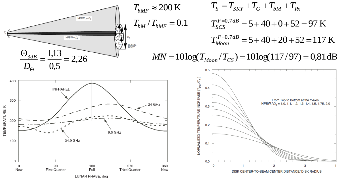
Obr. 9. Výpočet příspěvku šumu Měsíce pro anténu s aperturou 1,8 m.
