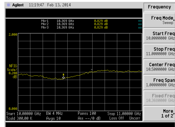
Obr. 8. LNA s vlnododovým vstupem. Šumové číslo bylo změřeno s přechodkou WR75/SMA (0,08 dB).
