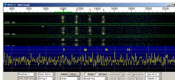
Obr. 5. Záznam signálu a komunikace EME módem JT4F se stanici ve Všenorech OK1KIR.
