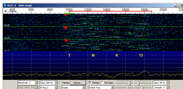
Obr. 6. Záznam signálu a komunikace EME módem QRA64D se stanici v Anglii G3WDG
