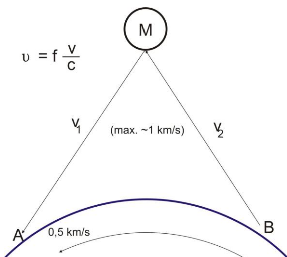
Obr. 3. Dopplerův posuv.
