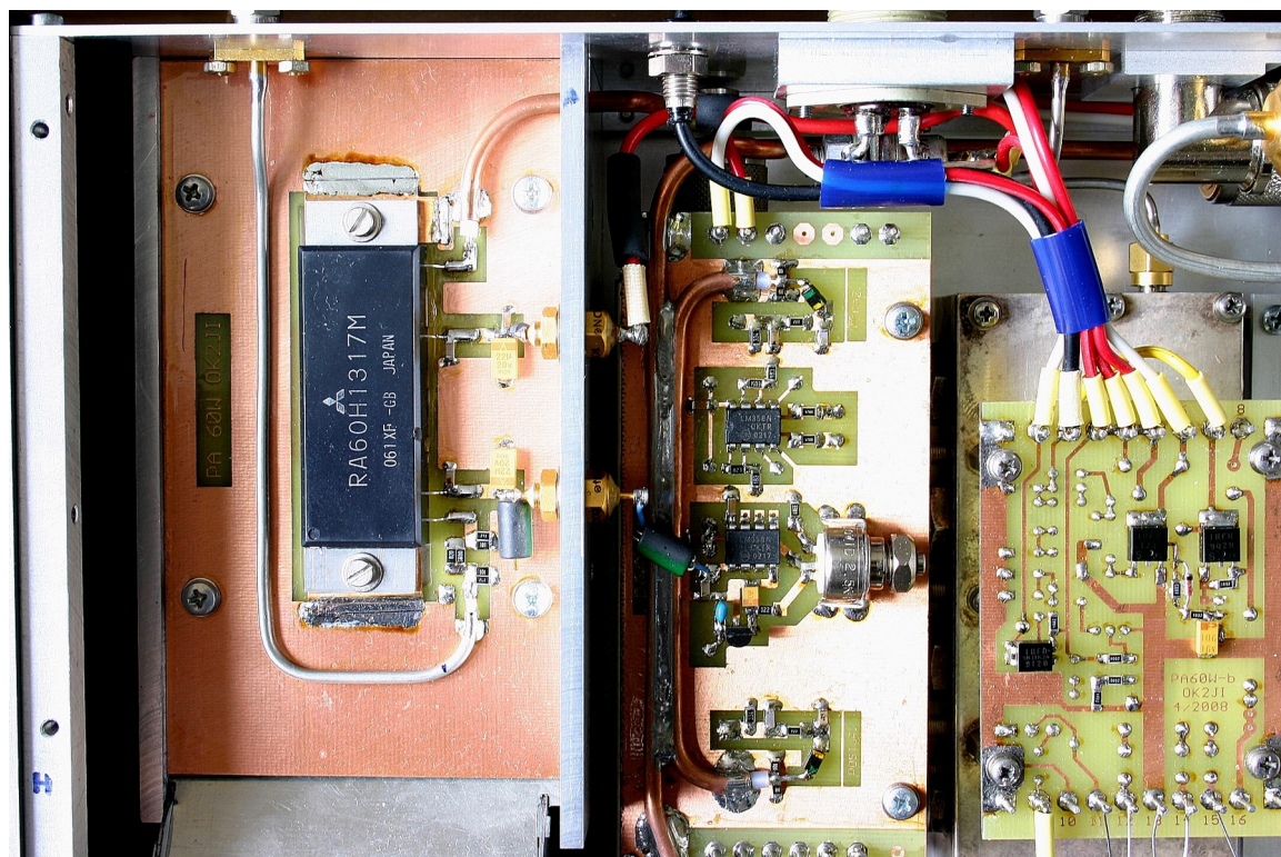
- 10 - Pohled na desku plošného spoje s mosfetovým modulem v bloku chladiče.
