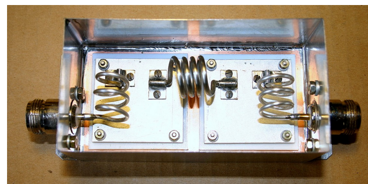
Detail výstupního filtru koncového stupně
