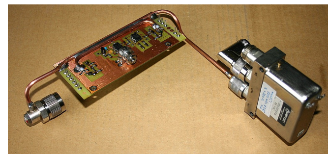
Deska s obvody reflektometrické ochrany PA
