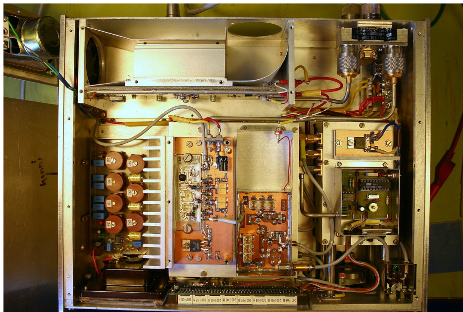
- 11 - Pohled do odkrytovaného TRXu zdola, vpravo je vidět mechanika chladícího tunelu s ventilátorem v levé bočnici bez PA.
