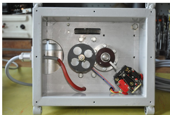
Transvertory pro 1296 a 2300MHz ve spojení se čtyřnásobnými anténami SBF. Jako mf. pro tato pásma je používán TRX-11 (foto již bylo uvedeno).
