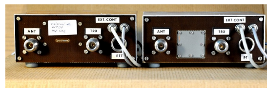
- 12 - Pro otáčení 12m stožáru zhotoven rotátor, na snímku vpravo je PA 30 W pro TRX11. Dále předzesilovače 144/432 MHz a RX- 432MHz.
