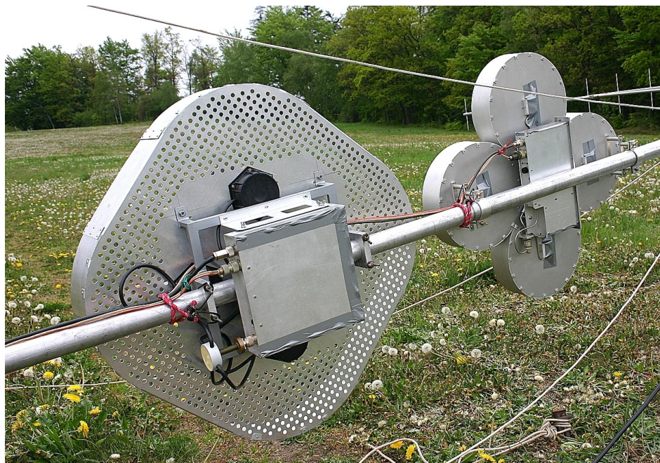
Transvertory pro 1296 a 2300MHz ve spojení se čtyřnásobnými anténami SBF. Jako mf. pro tato pásma je používán TRX-11 (foto již bylo uvedeno).
