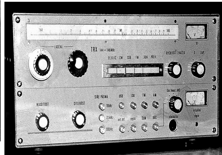
První TRX s výkonem asi 5W byl zhotoven pro OK1KRG
