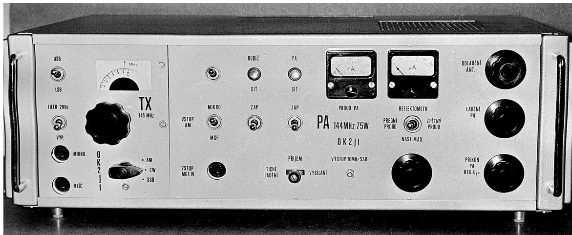
První, větší laditelný SSB TX pro 144MHz používaný pro závody a provoz přes satelit „OSCAR-6“: Zařízení bylo realizováno asi v roce 1971.
