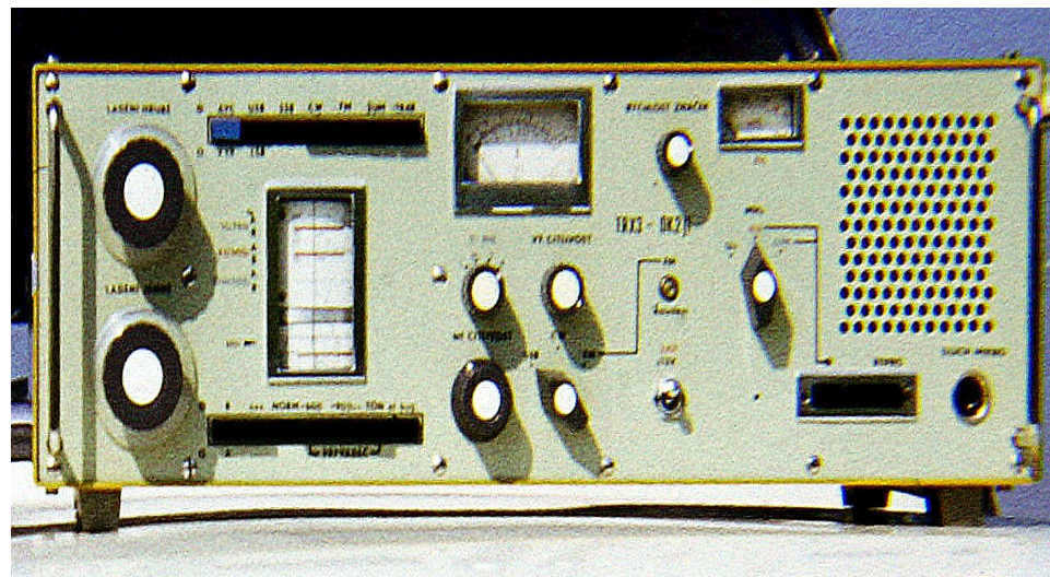
TRX-3 pro 432MHz, použitý v soutěži VKV-34 a VKV-35 (SSSR a NDR).
