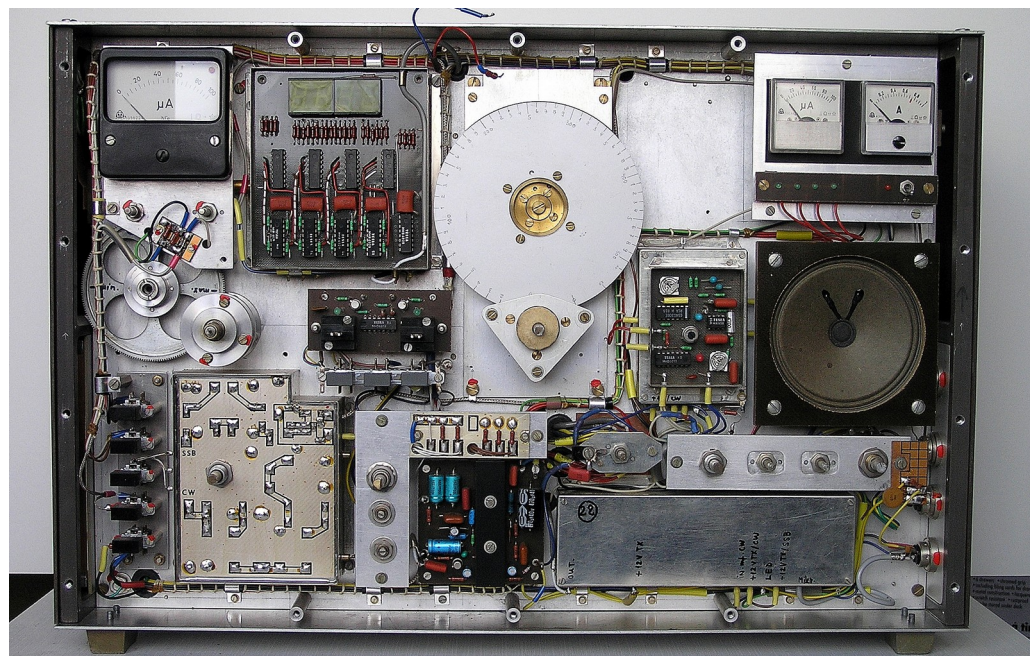
TRX-8 po sejmutí čelního panelu. Zařízení má dva samostatné oscilátory
