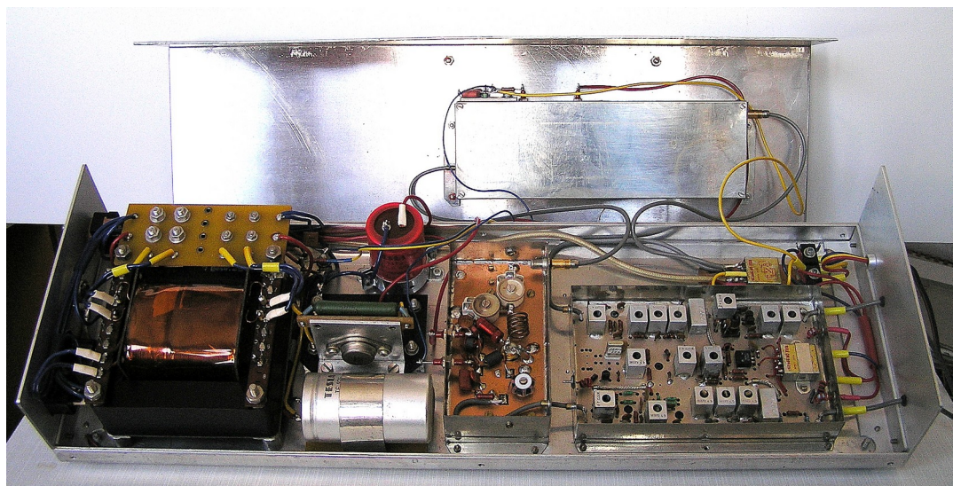
- 7 - Transvertor 50MHz pro TRX-8 s výkonem 10W.
