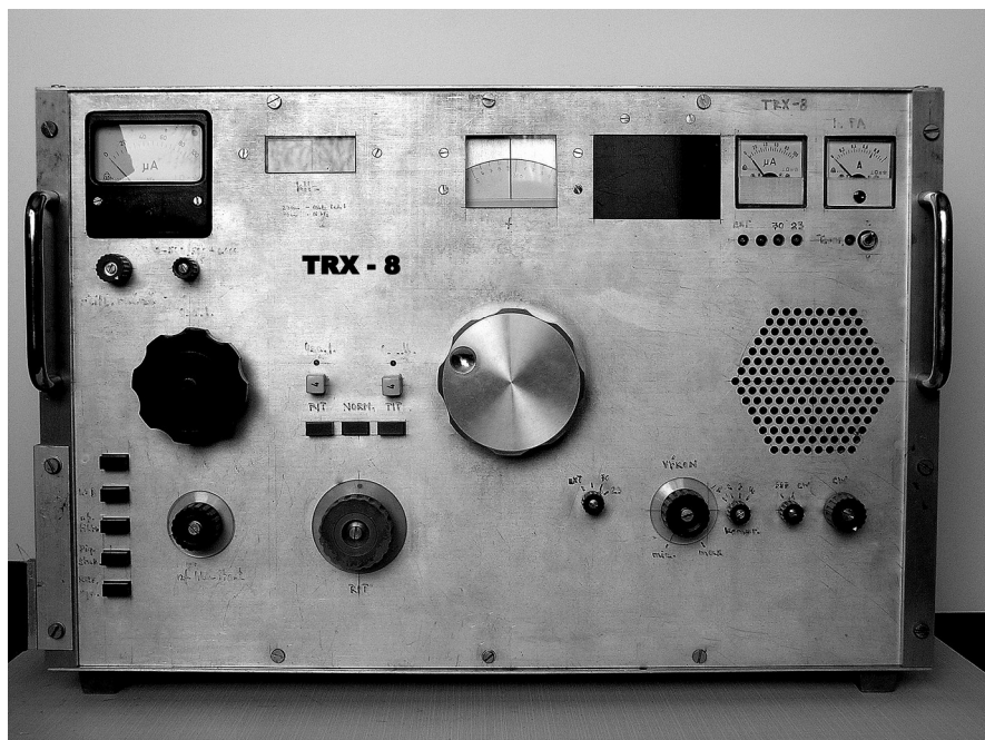
TRX-8 432, 1296MHz a jako mf. pro transvertor na pásmo 50MHz
