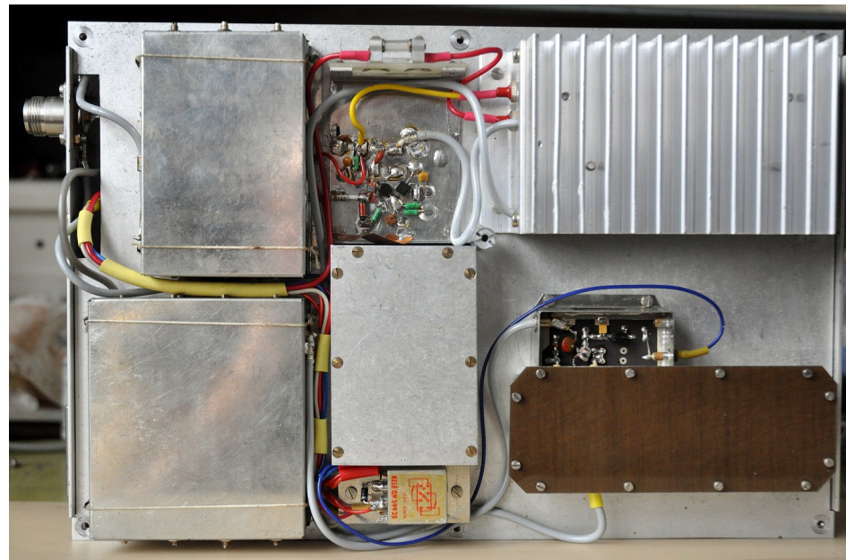
Pohled do TRX-10 po sejmutí krytu na mechanické a elektrické díly zařízení, vedlejší obrázek ukazuje chladič PA a budící stupně TXu včetně ant. Relé.
