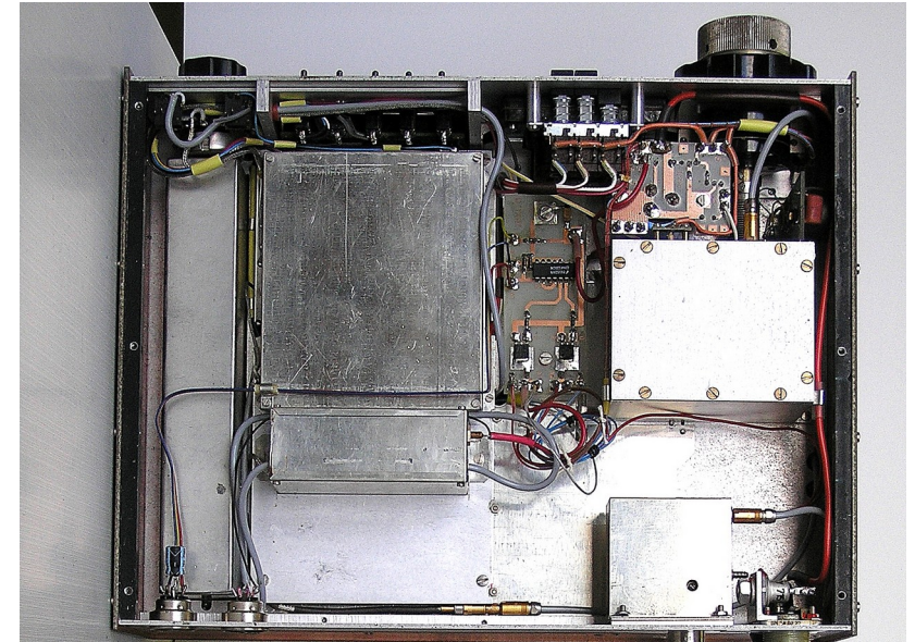
TRX-11 Zařízení pro 144Mhz a transvertory 1296/2300Mhz out. 100mW V zařízení použit Xtalový 14ti násobný příčkový filtr. (patrný na snímku vpravo)
