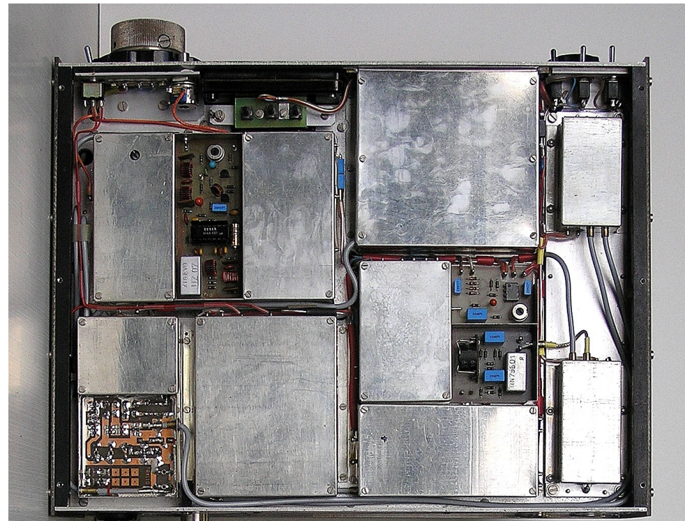
TRX-11 Zařízení pro 144Mhz a transvertory 1296/2300Mhz out. 100mW V zařízení použit Xtalový 14ti násobný příčkový filtr. (patrný na snímku vpravo)
